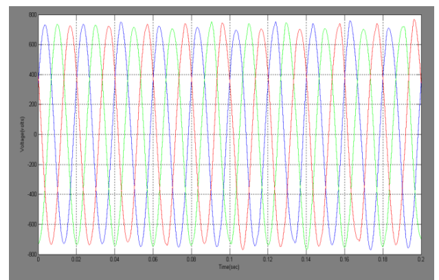
(d) Three phase voltage
